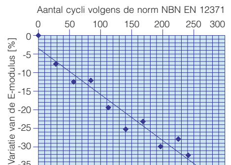
Afb. 2 Verlies aan mechanische sterkte door vorst-dooicycli zonder zichtbare schade.
